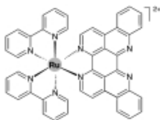
\Lambda -[Ru(bpy) 2 (eilatrin)] 2+
