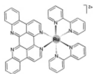
\Delta -[Ru(bpy) 2 (eilatrin)] 2+
